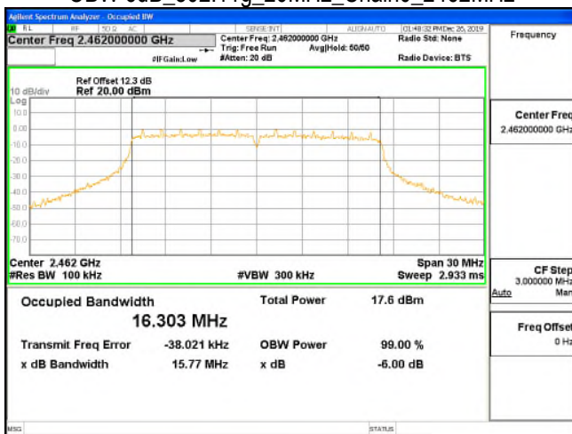
OBW 6dB_802.11g_20MHz_Chain0_2462MHz
