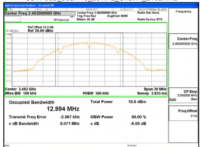
OBW 6dB_802.11b_20MHz_Chain1_2462MHz
