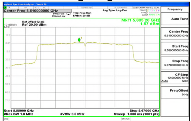
802.11ac_80MHz_5610MHz
