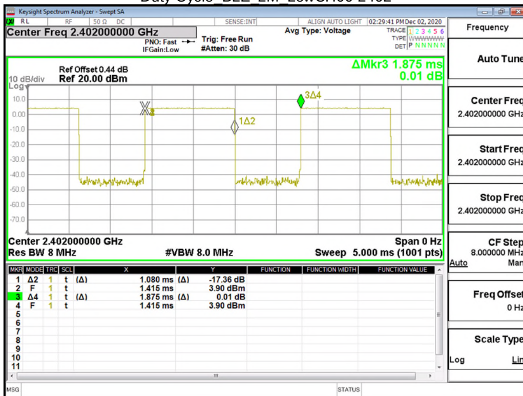
Duty Cycle BLE 2M LowCH00-2402
