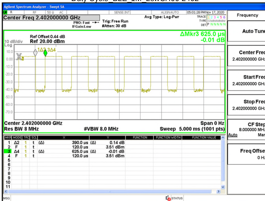
Duty Cycle BLE 1M LowCH00-2402
