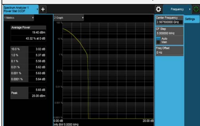
64QAM CH 21425 (2567.5MHz)
