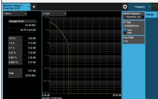
64QAM CH 20350 (1750MHz)
