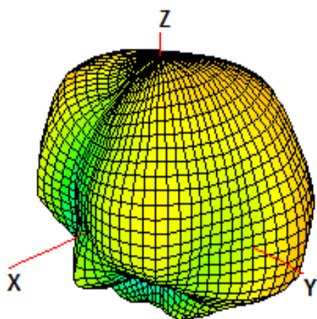
5150MHz ANT4
