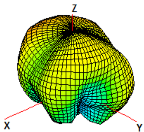
5850MHz ANT4
