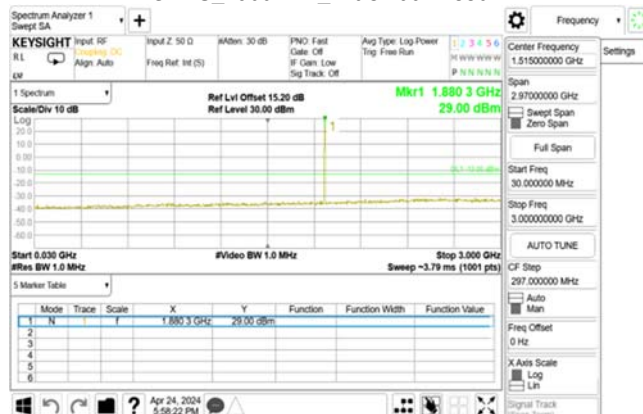
GPRS_1900MHz_MidCH661-1880
