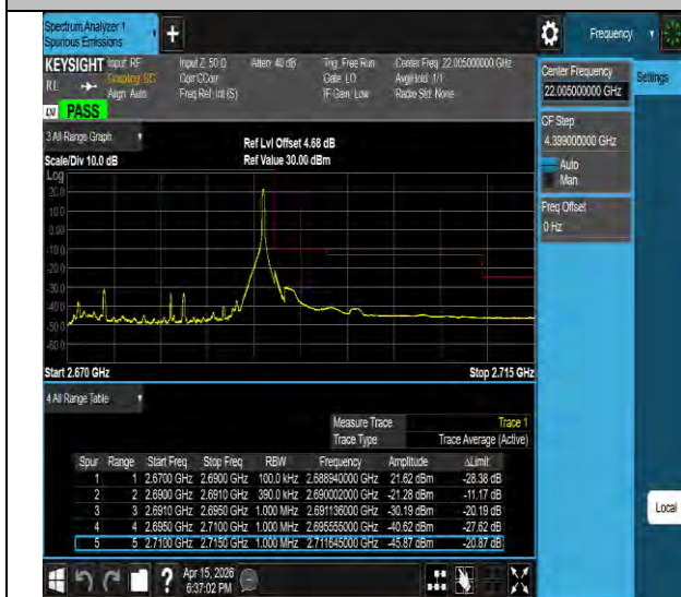
Band41-20MHz-QPSK-41490-1RB#99-PASS
