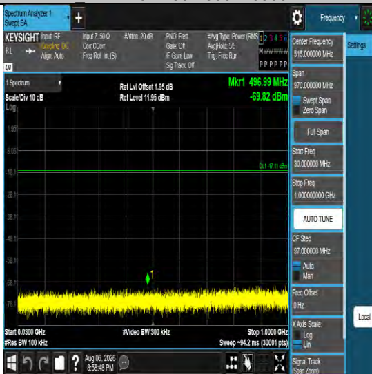
BLE 2M-Ant6-2402-30~1000-PASS
