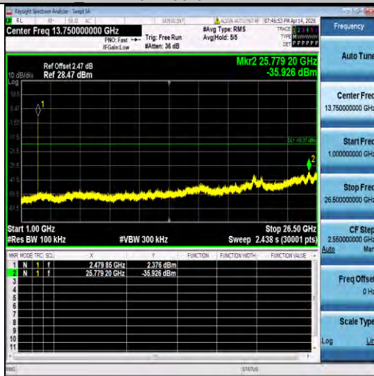
BLE 1M-Ant6-2480-1000~26500-PASS
