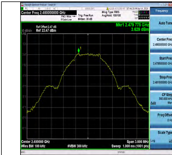
BLE 1M-Ant6-2480-0~Reference-PASS
