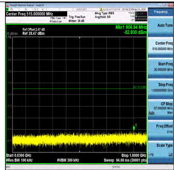
BLE 1M-Ant6-2480-30~1000-PASS
