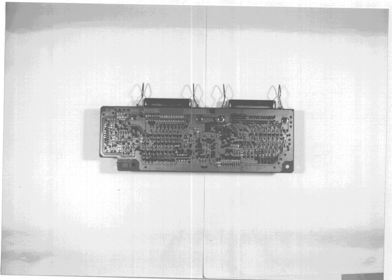
Photo - 2 : AL-8PK : Interface PWB ( 2 / 2 )
