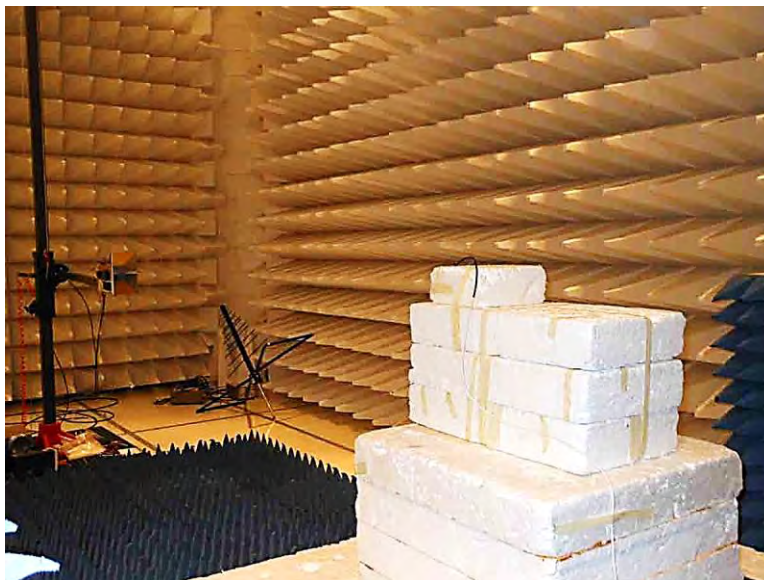
Configuration 1, 1 – 12GHz
