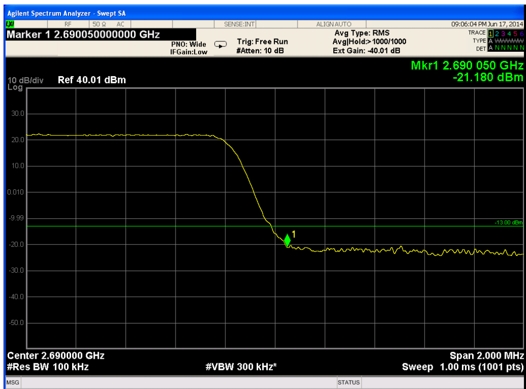
Figure 204.— 2687.50 MHz QPSK
