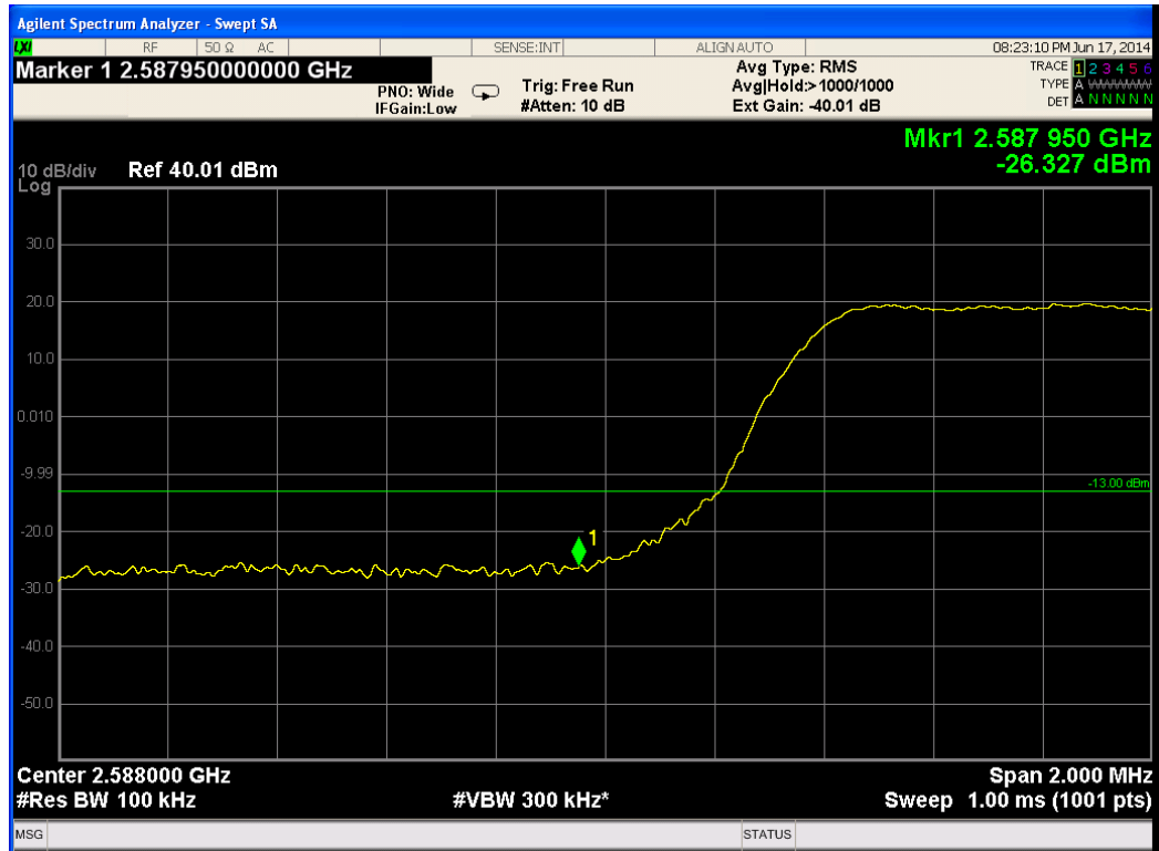
Figure 219.— 2593.00 MHz 64QAM
