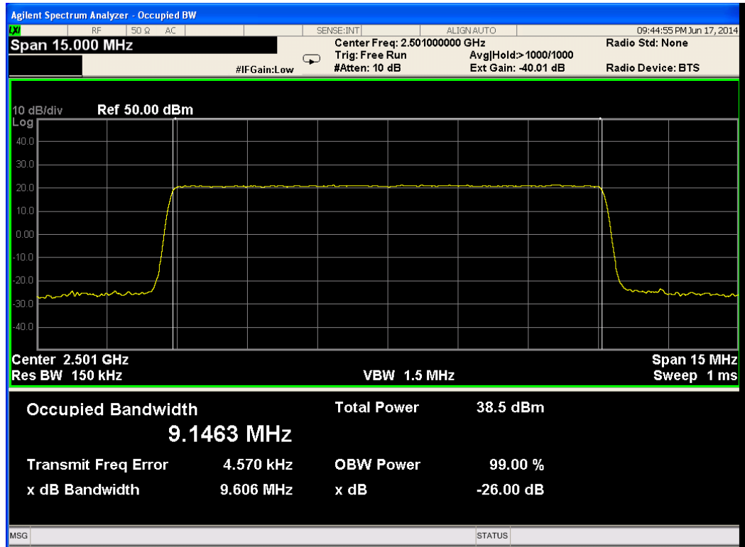
Figure 164.— 2501.00 MHz QPSK
