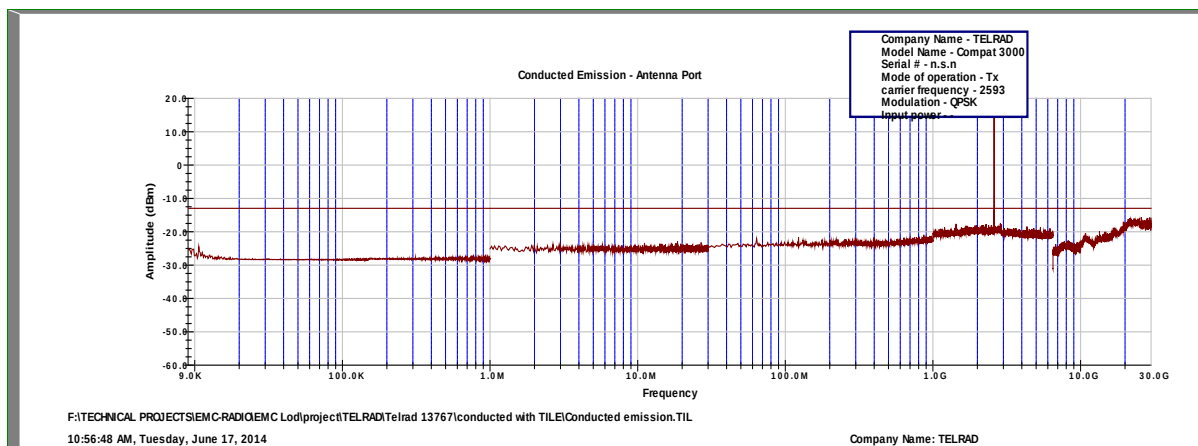
Figure 176.— 2593.00 MHz QPSK
