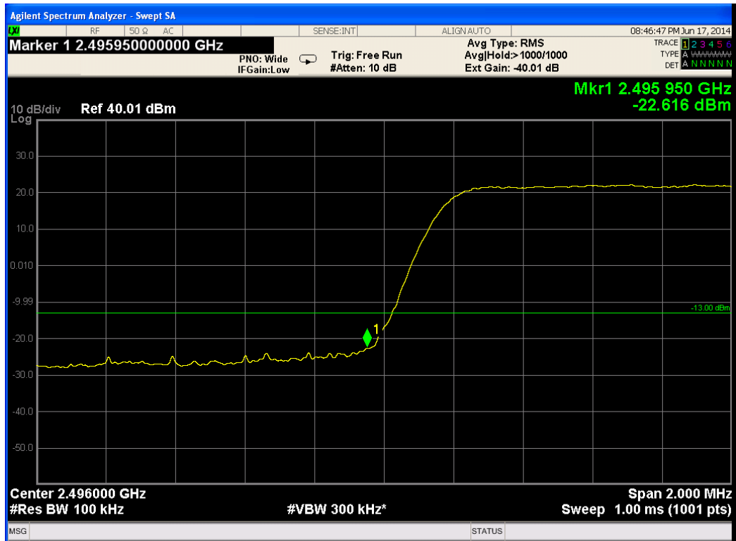
Figure 195.— 2498.50 MHz 64QAM
