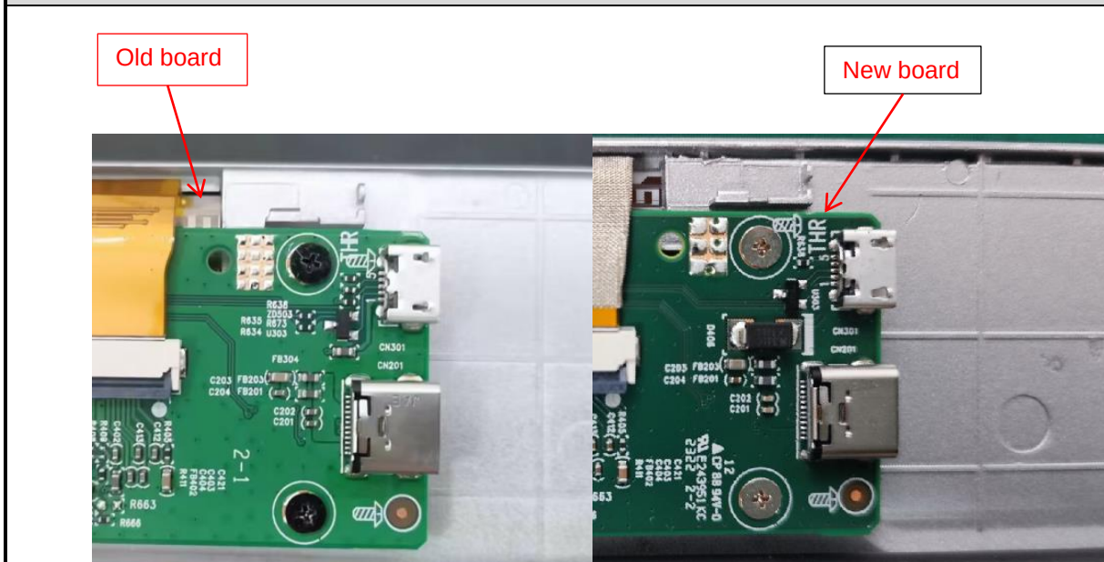
EUT Photo
