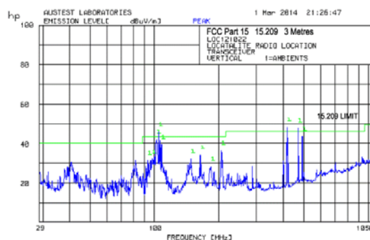
Vertical Polarisation
