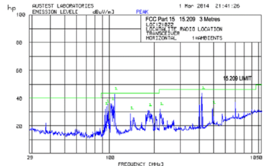
Horizontal Polarisation
