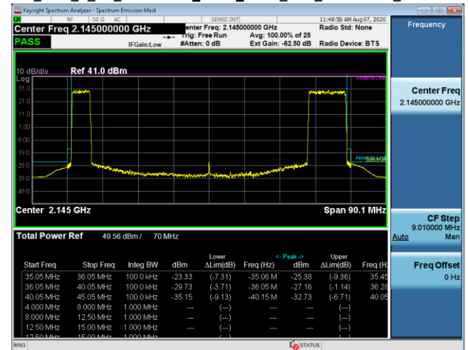
OOBE_TM3_1_2C_5+10MBW_2112_2175_TX1_33W+57W_LTE+5G-NR
