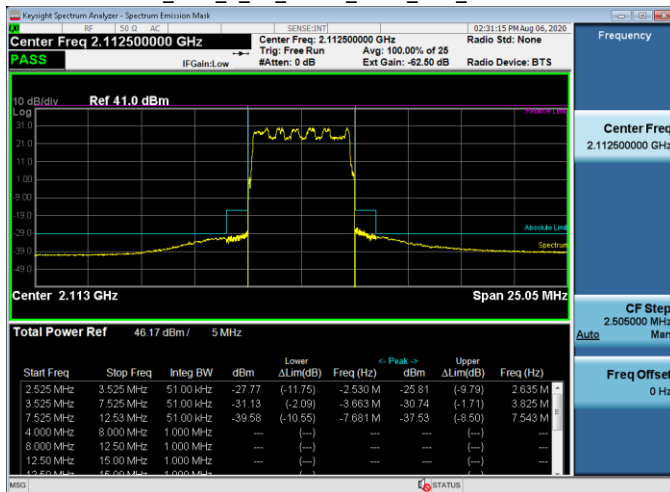
Oobe_TM3_2_1C_5MBW_2112_TX1_40W 5G-NR
