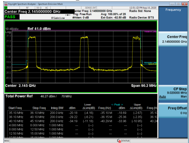
OOBE_TM3_2_3C_5+5+5MBW_2112_2145_2177_TX1 46W_LTE+LTE+5G-NR
