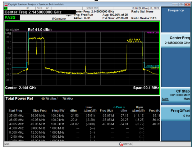
OOBE_TM3_2_3C_5+5+10MBW_2112_2117_2175_TX1 30W+30W+30W_LTE+LTE+5G-NR
