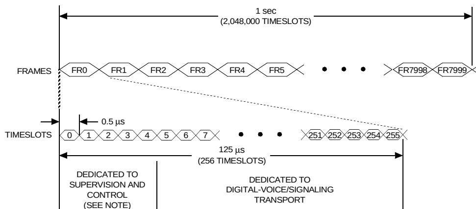
A. E1/CEPT TRANSMISSION FORMAT
