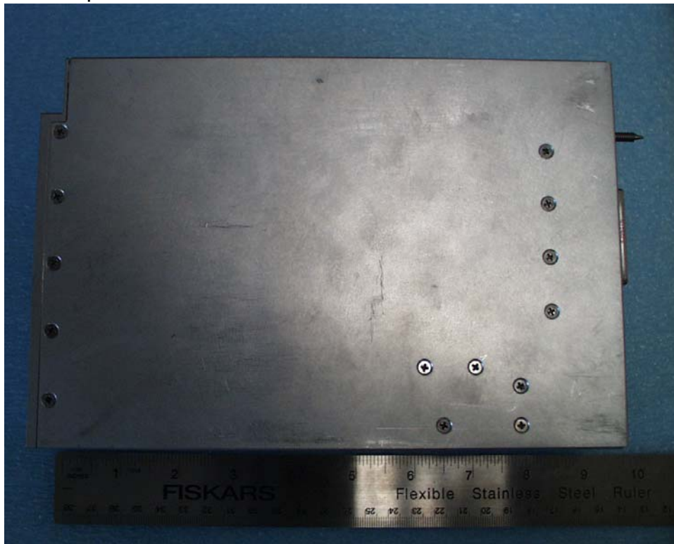
EUT Top
