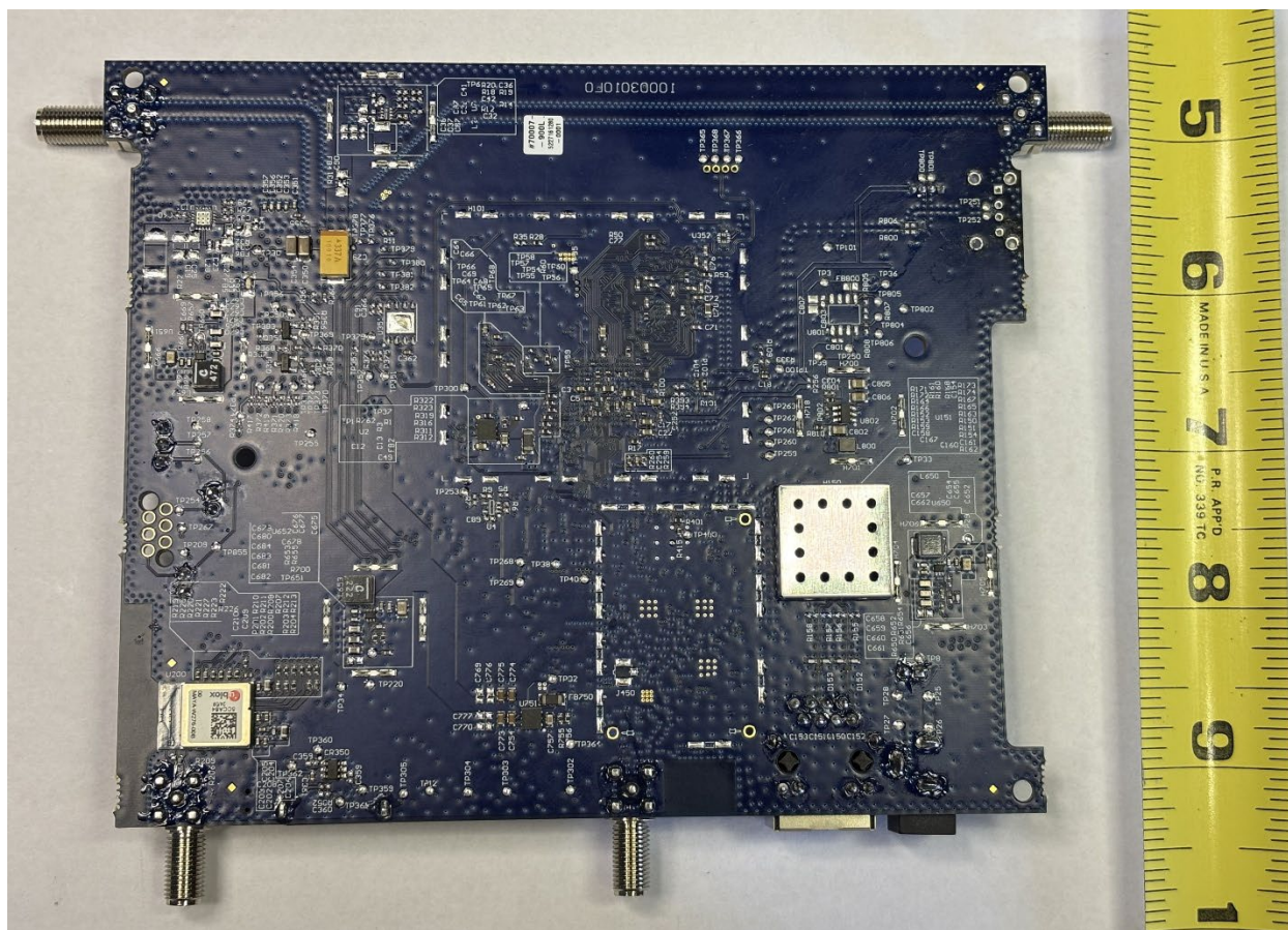
PCB Bottom
