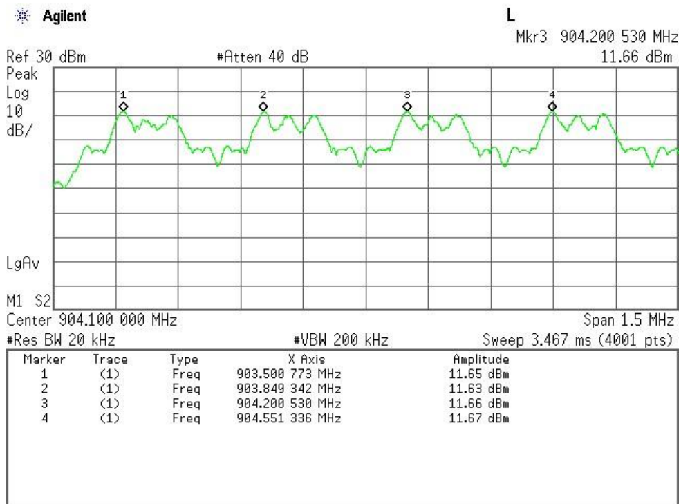
Channel 1-4 (Walkie-Talkie Mode)
