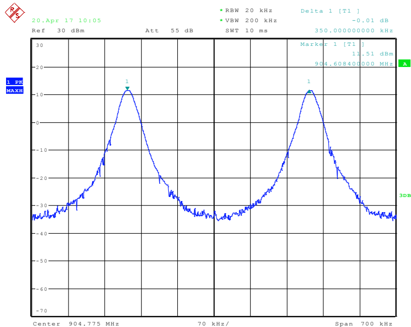
Channel 3 and 4 (Walkie Talkie)
