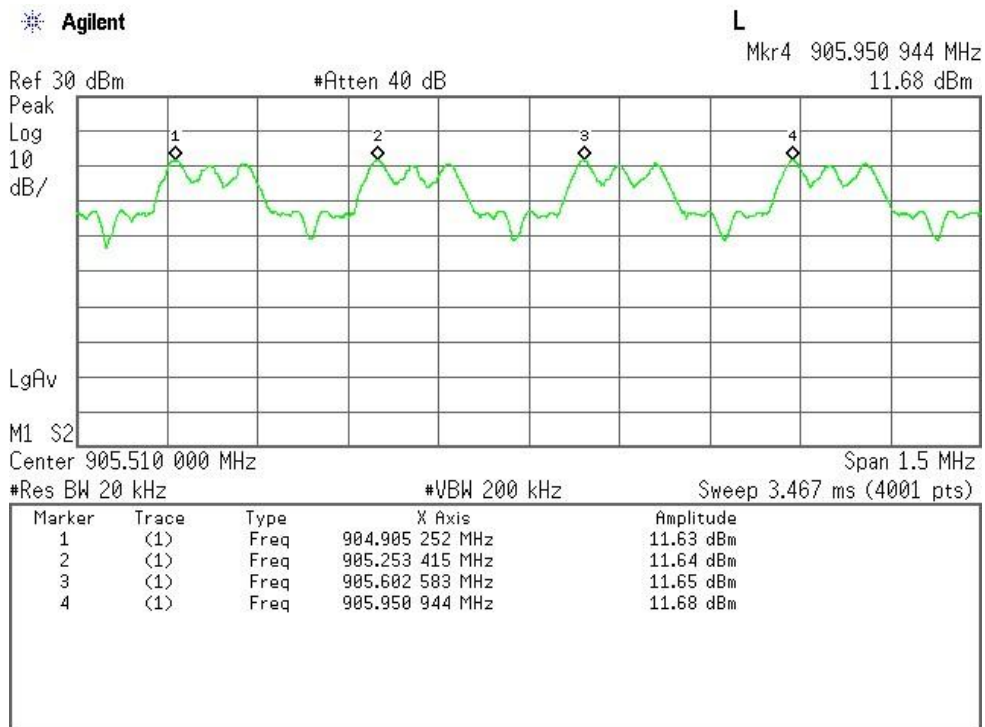
Channel 5-8 (Walkie-Talkie Mode)
