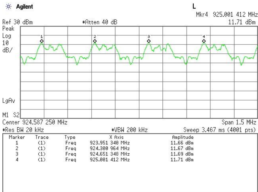
Channel 21-24 (Walkie-Talkie Mode)
