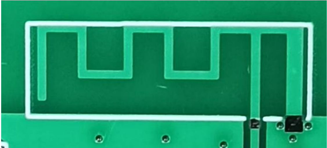
天线实物及物理尺寸
