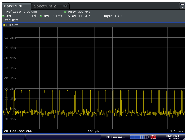
35 µs Pulses
