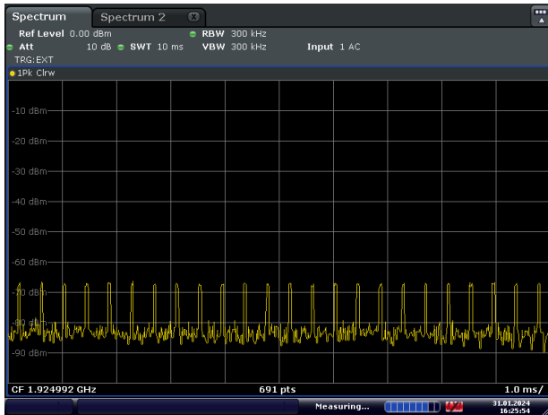
50 µs Pulses
