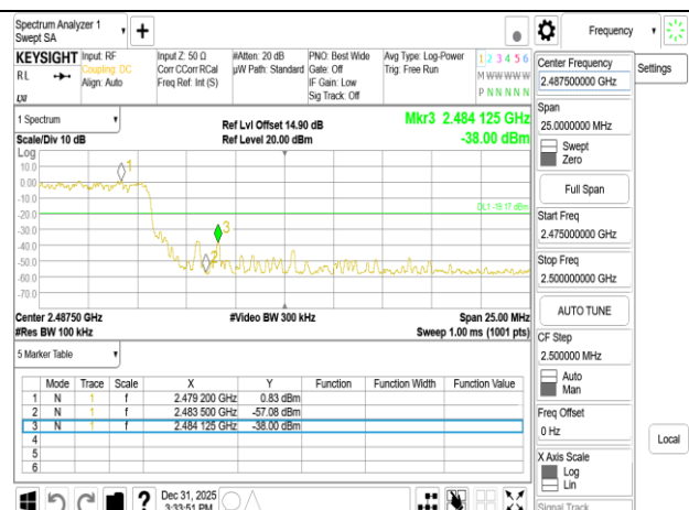
Hopping Band Edge 8DPSK 3M DH5 2480MHz
