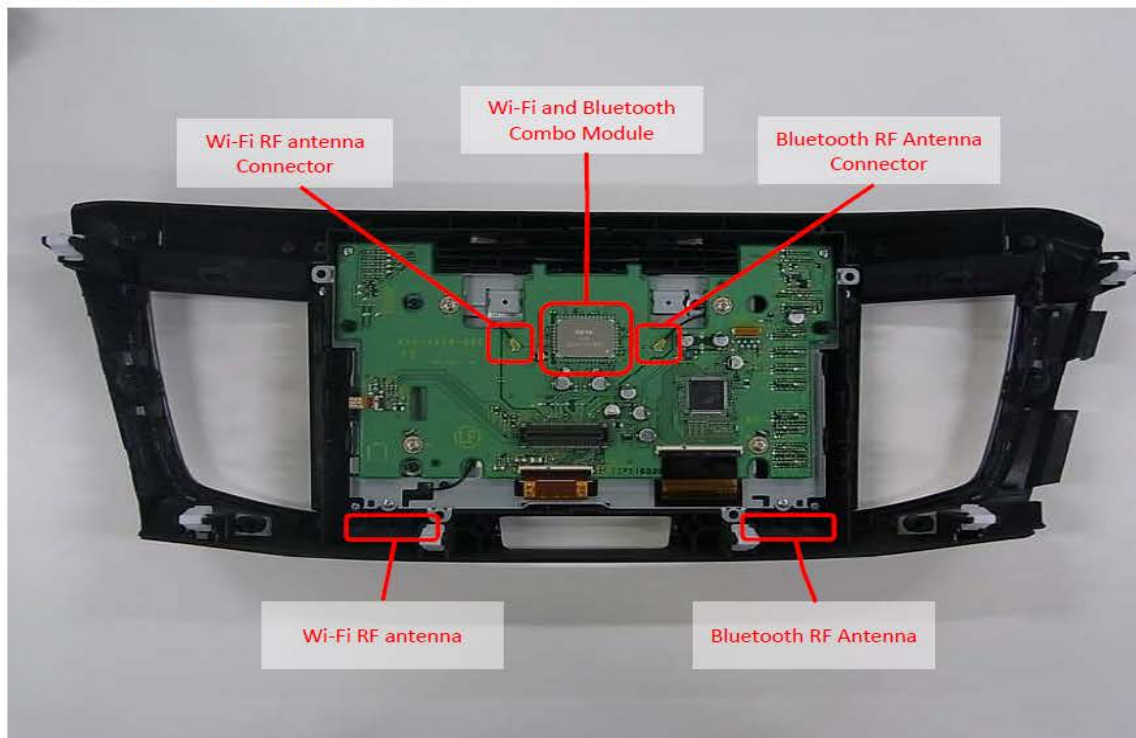
1-1. LCD PCB ASSY Component - F1 View
