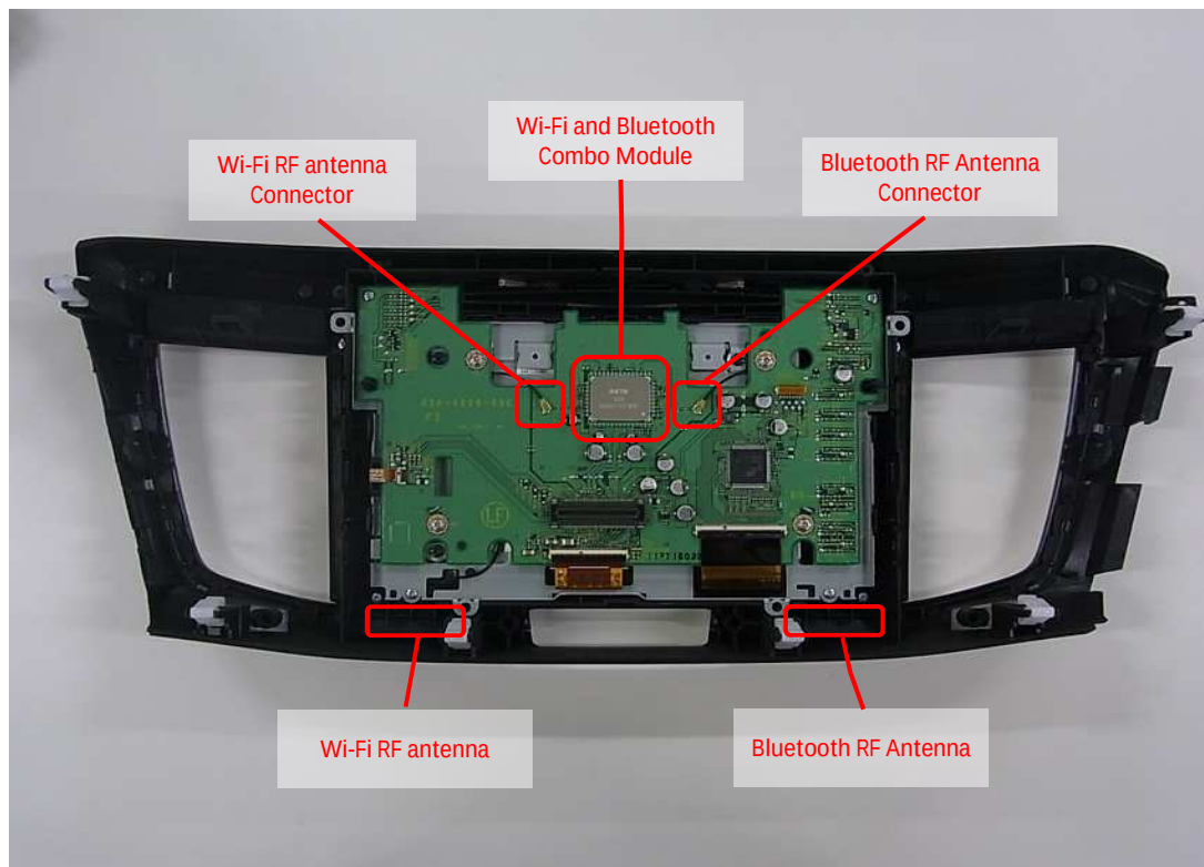
1-1. LCD PCB ASSY Component - F1 View
