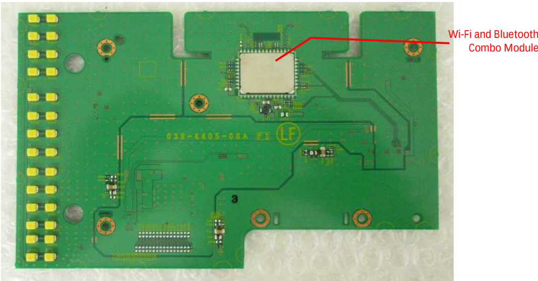
LCD PCB ASSY - F1 View
