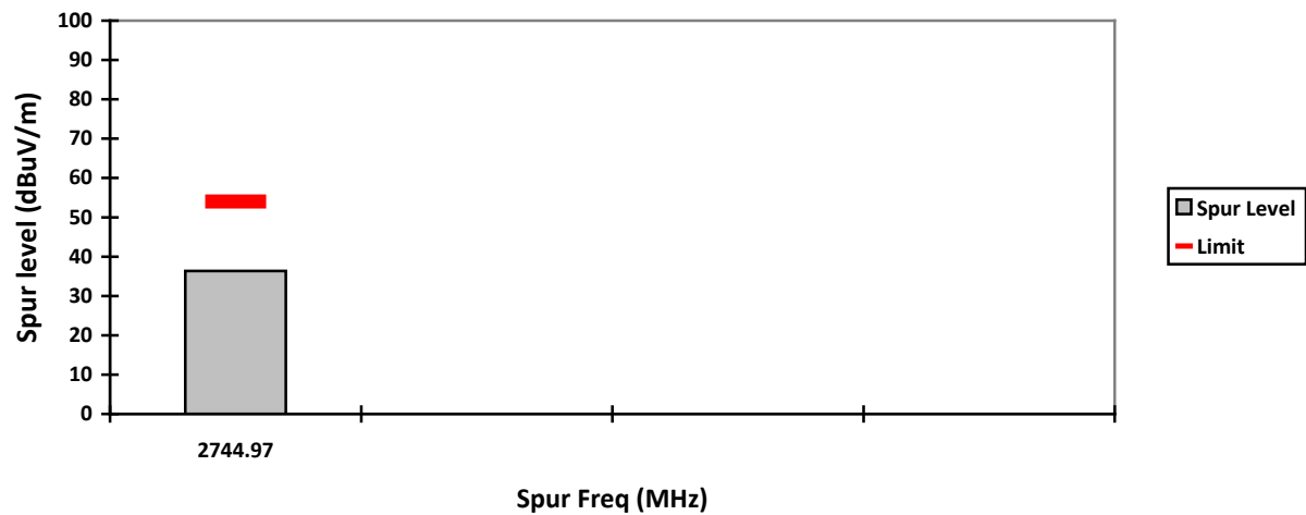
VERTICAL, AV
