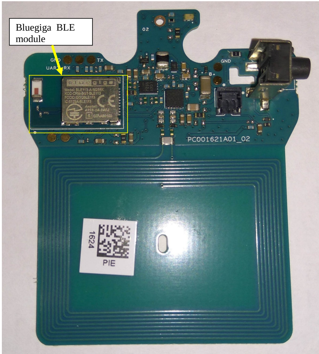
PCB Top
