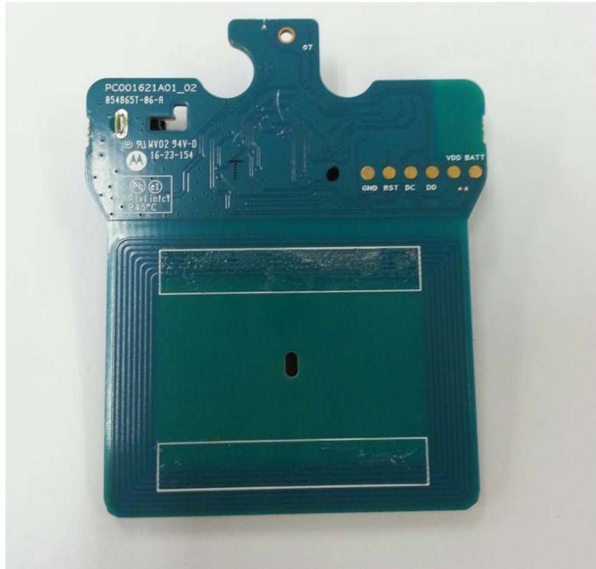
PCB Bottom
