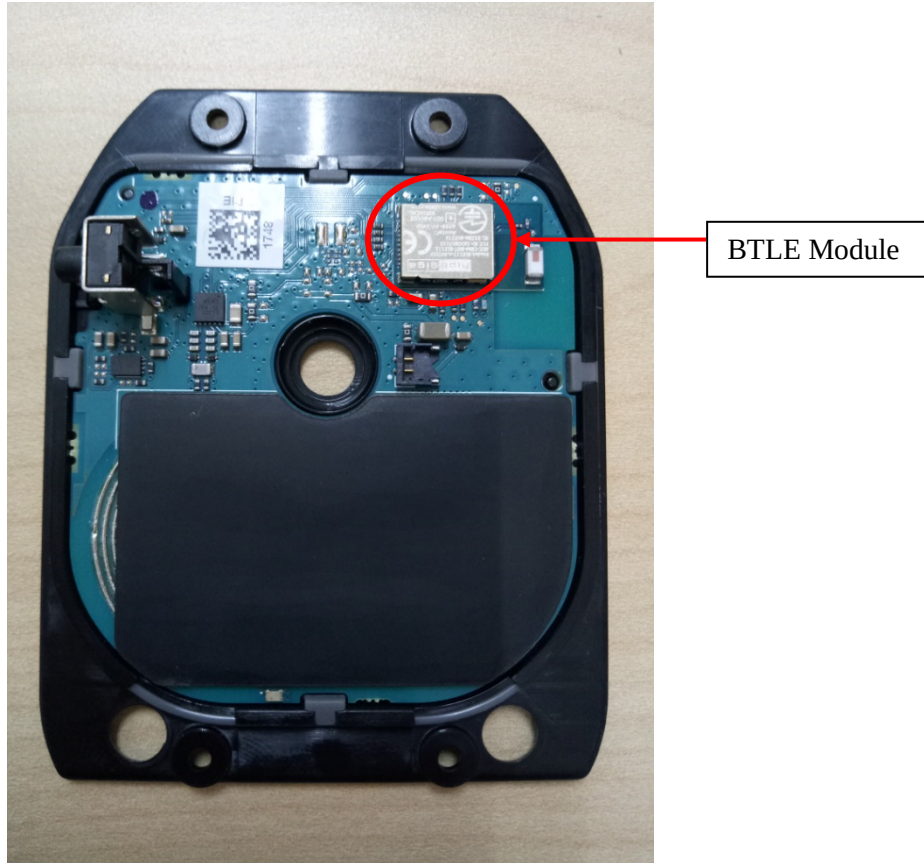
PCB Top
