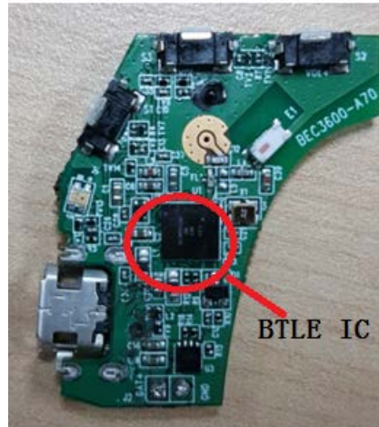
PCB Top
