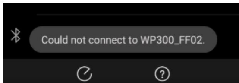
Abbildung 1 : Meldung
