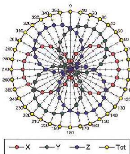
f = 100 \text{ MHz} , TEM cell ifi110
