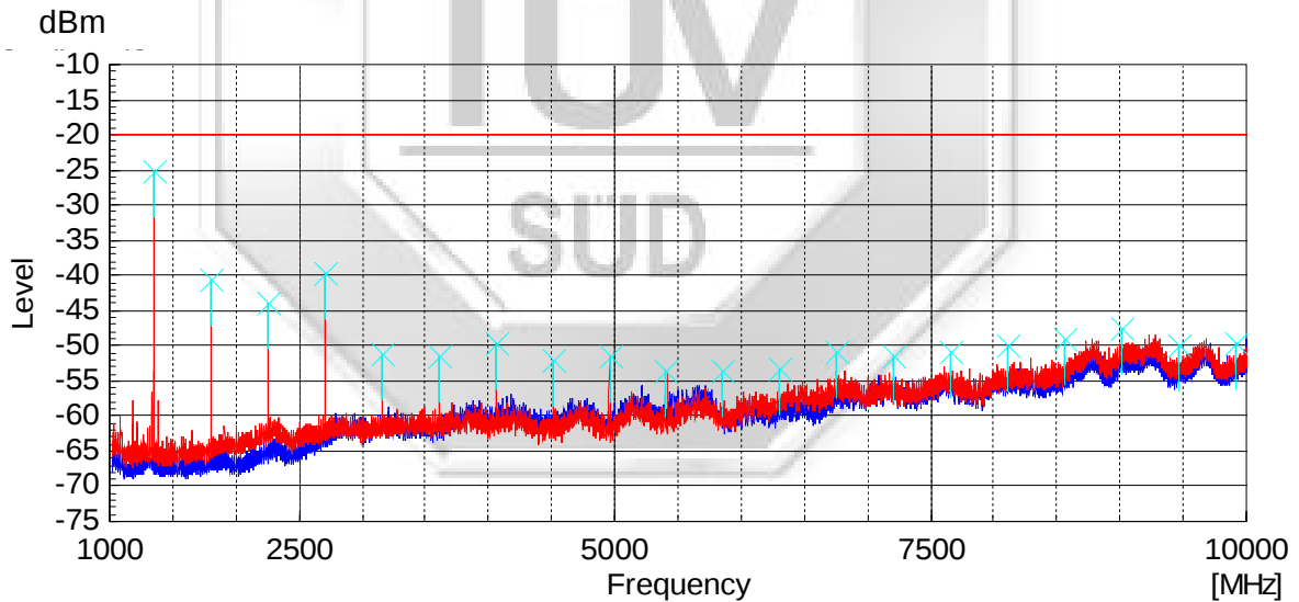
450.65MHz (Digital) 1GHz - 10GHz
