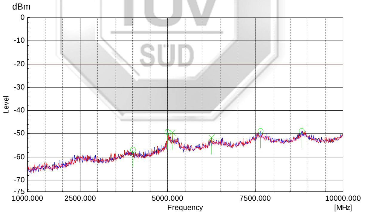
450.65MHz (Digital) 1GHz – 10GHz
