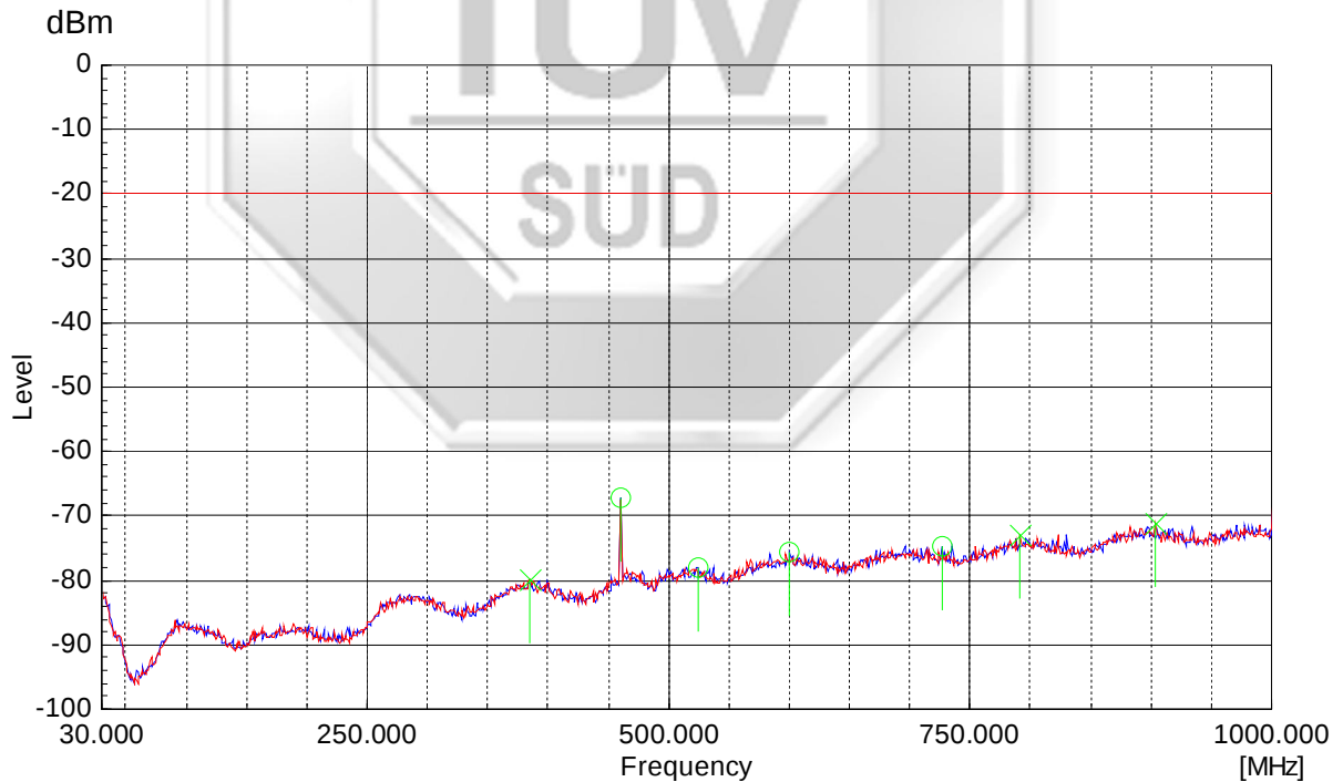
459.125MHz (Digital) 30MHz – 1GHz
