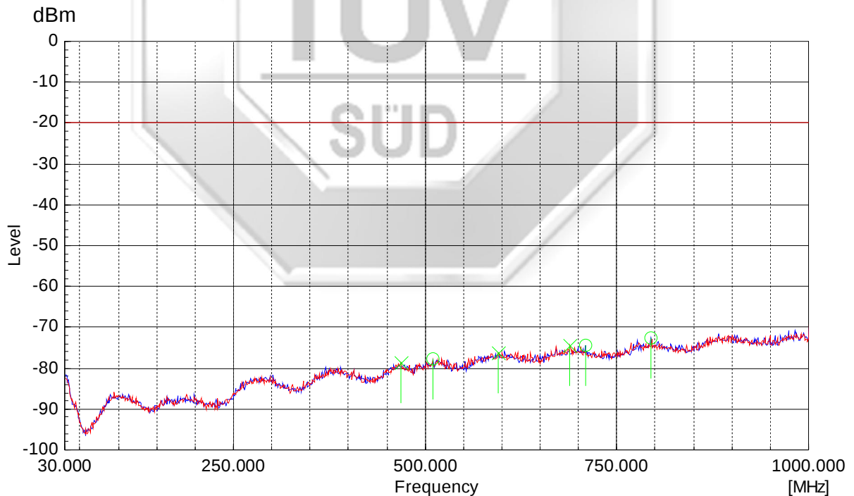
406.2MHz (Digital) 30MHz – 1GHz
