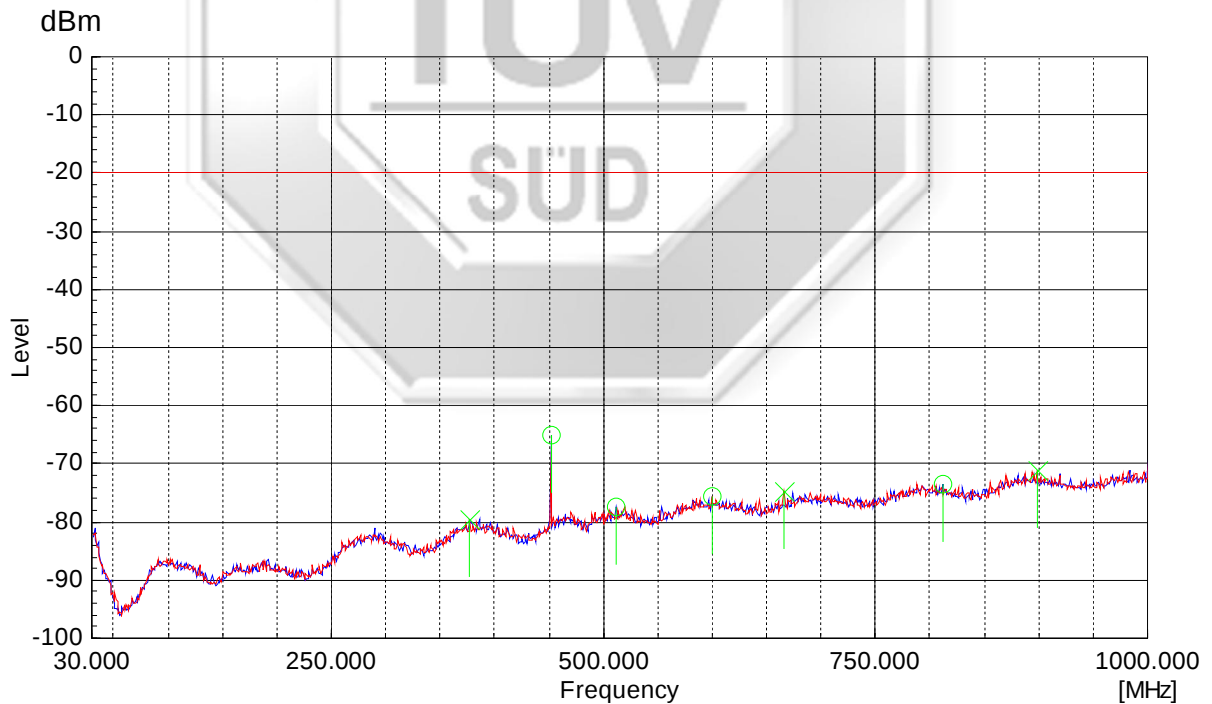
450.65MHz (Digital) 30MHz – 1GHz
