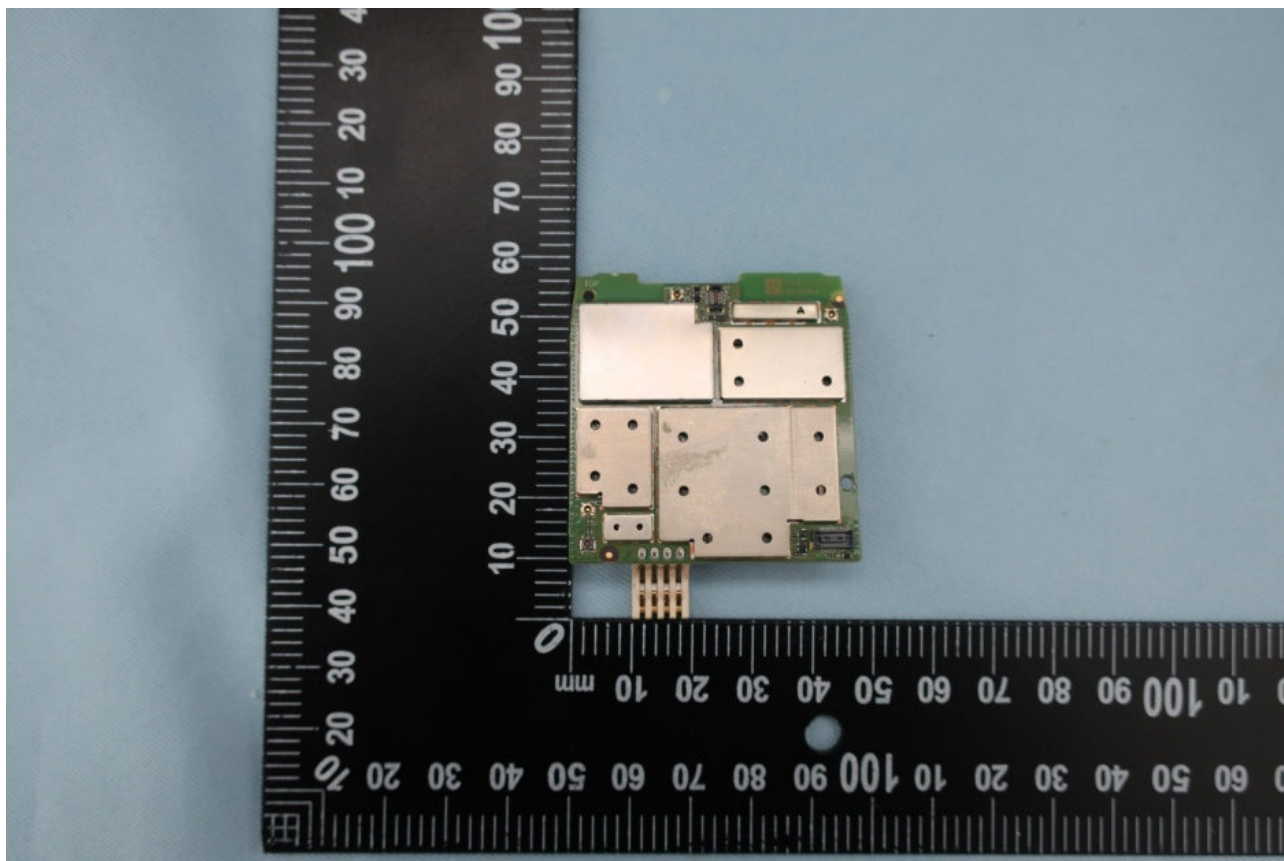
<Main PCBA bottom side>
