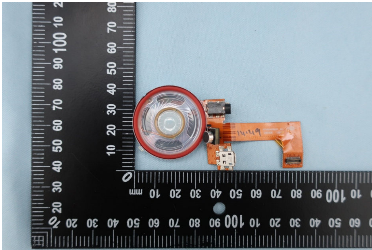
<Speaker_mic_USB_audiojack FPCA top side>
