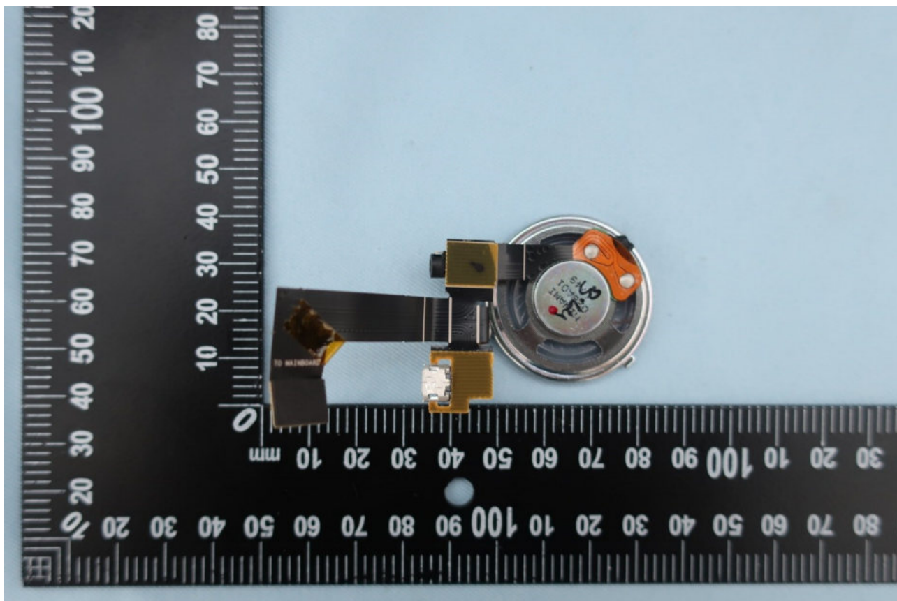
<Speaker_mic_USB_audiojack FPCA bottom side>
