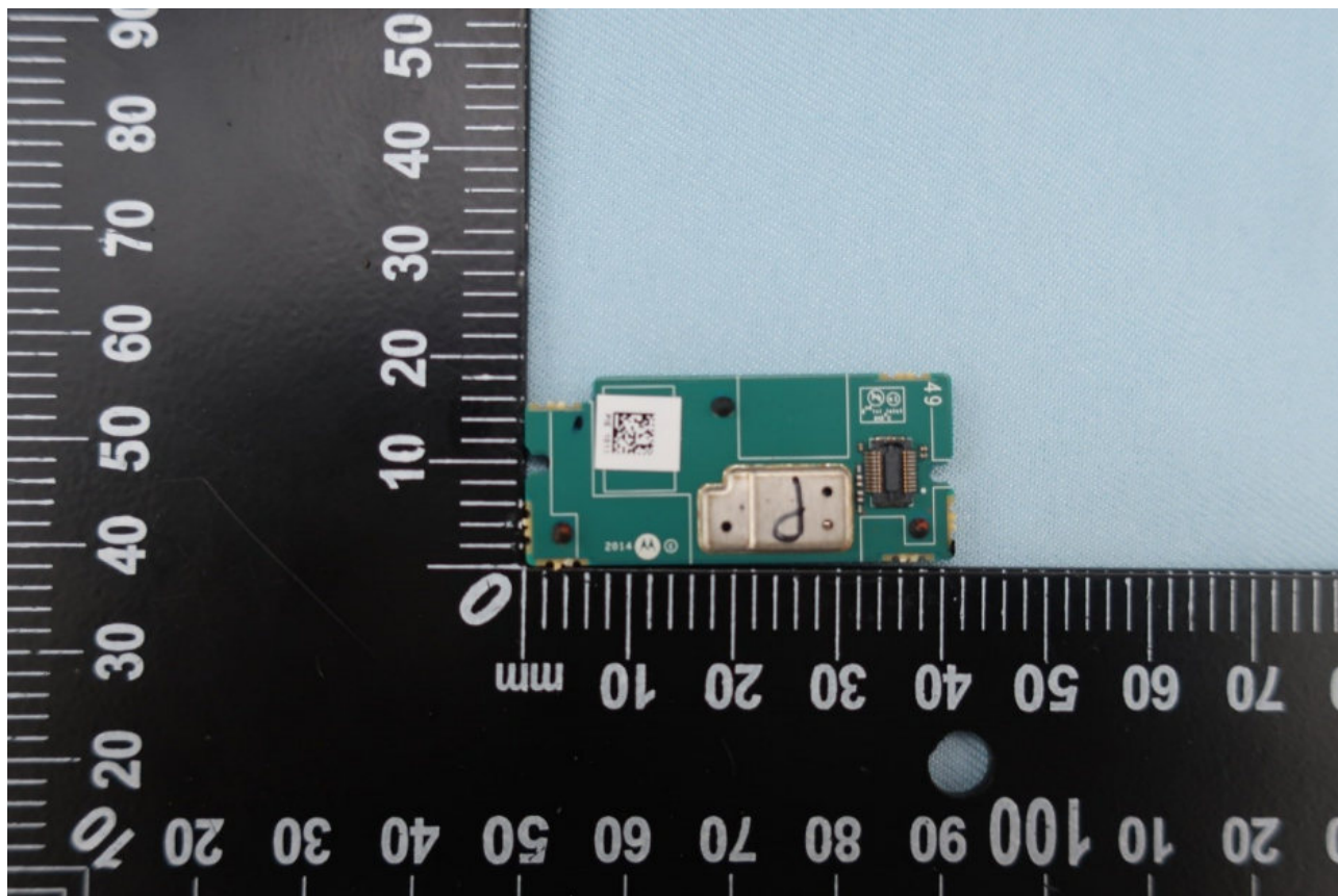
<Display PCBA bottom side>
