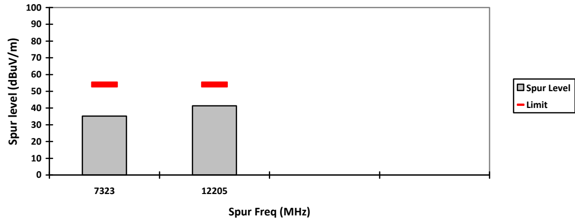
VERTICAL, AV
