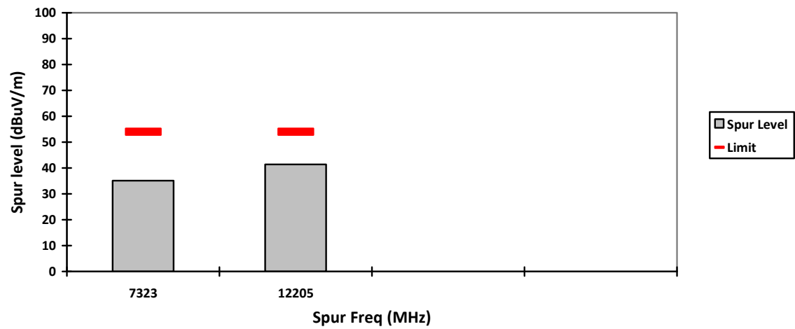
HORIZONTAL, AV
