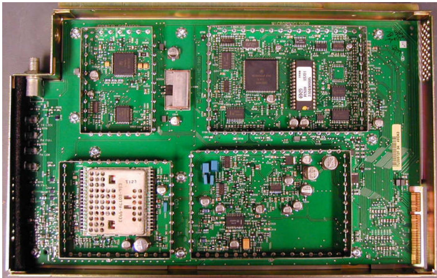
EXCITER MODULE
