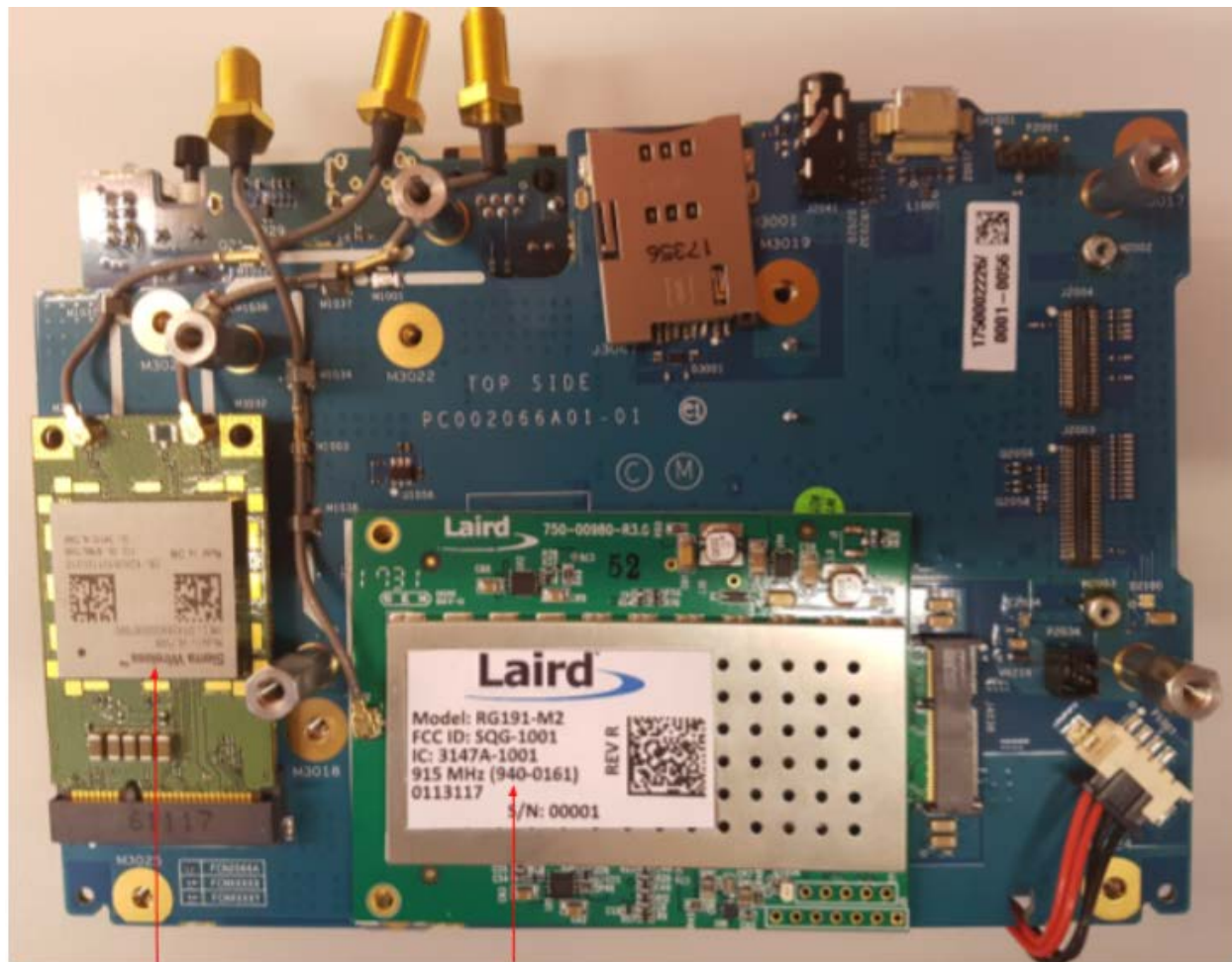
LTE Module
