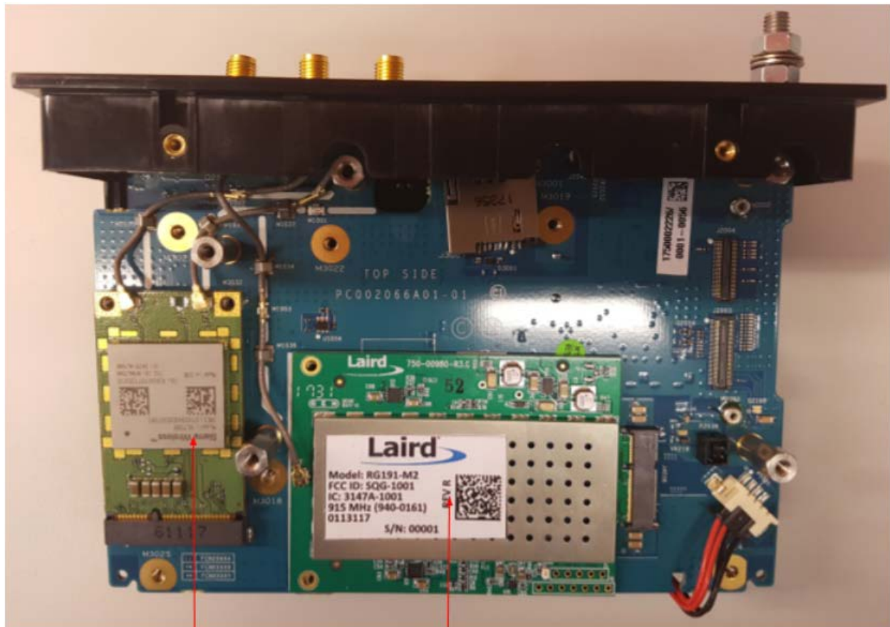
LTE Module
