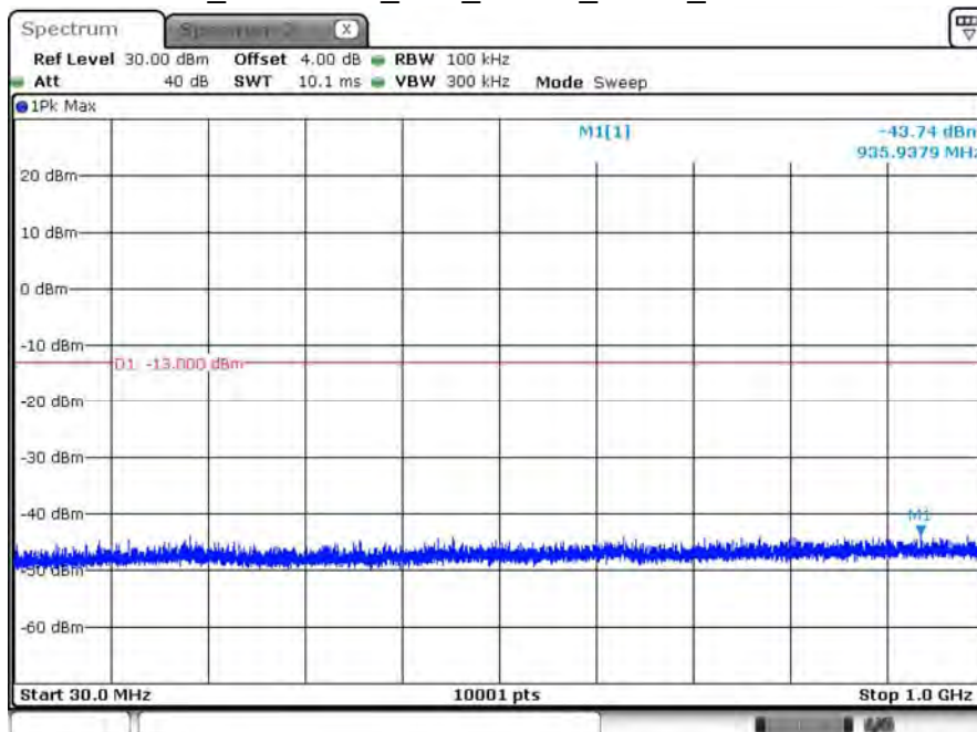
B66_CH132572_20M_1RB49_QPSK_Below 1G
