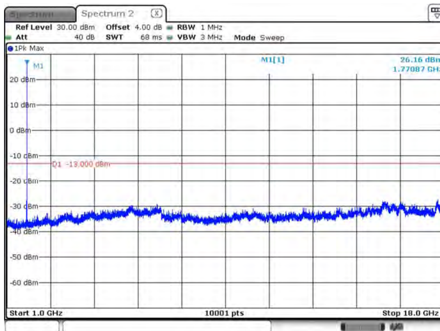
B66_CH132572_20M_1RB49_QPSK_Above 1G
