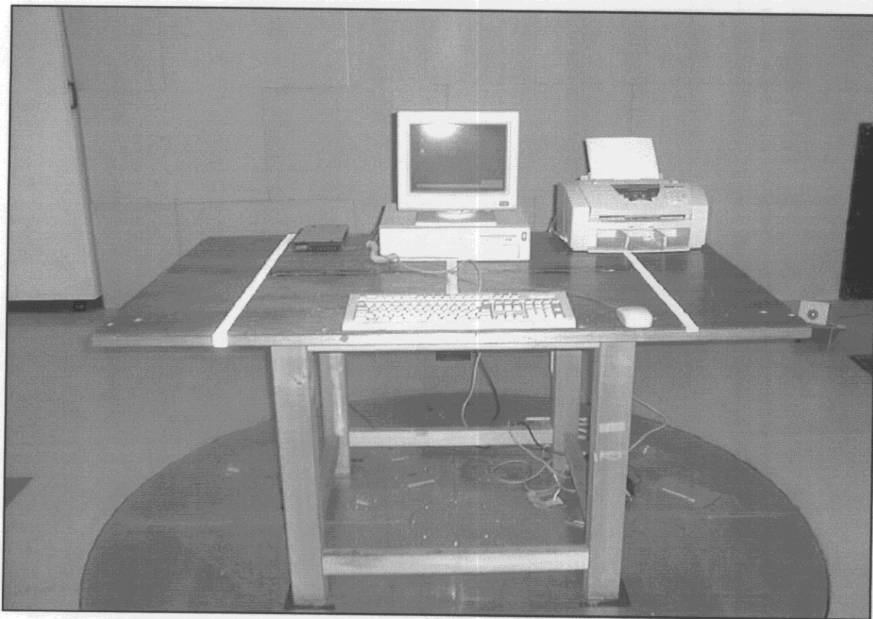
正面(放射ノイズ測定時) Front View (Radiation)
