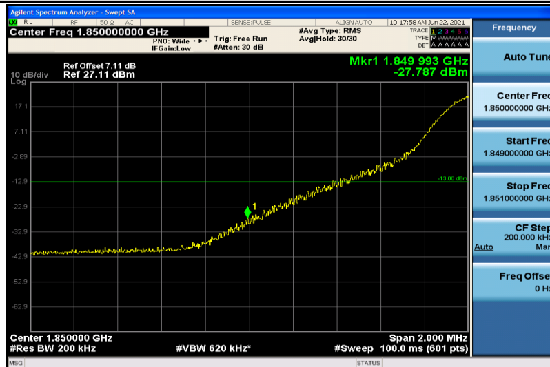
Band25-20MHz-QPSK-26140-1RB#0
