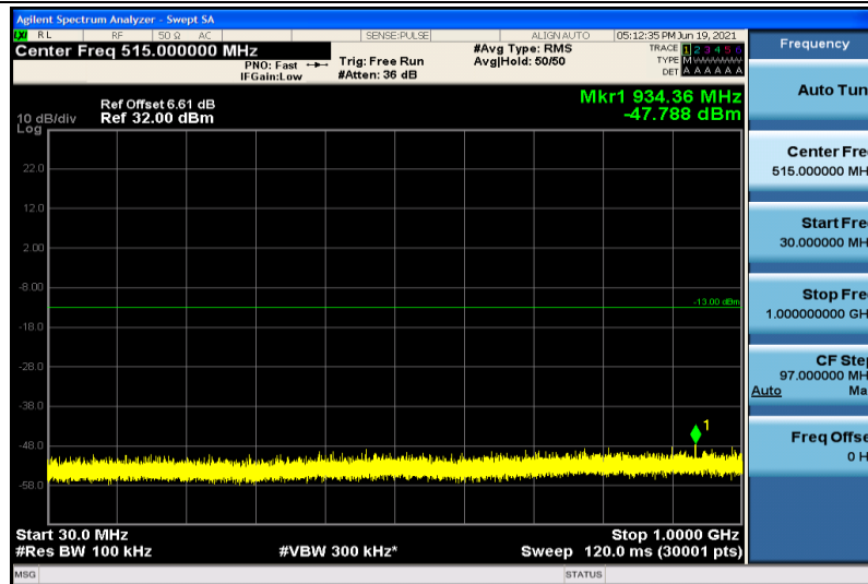
Band25-20MHz-16QAM-26365-1RB#0-30~1000MHz
