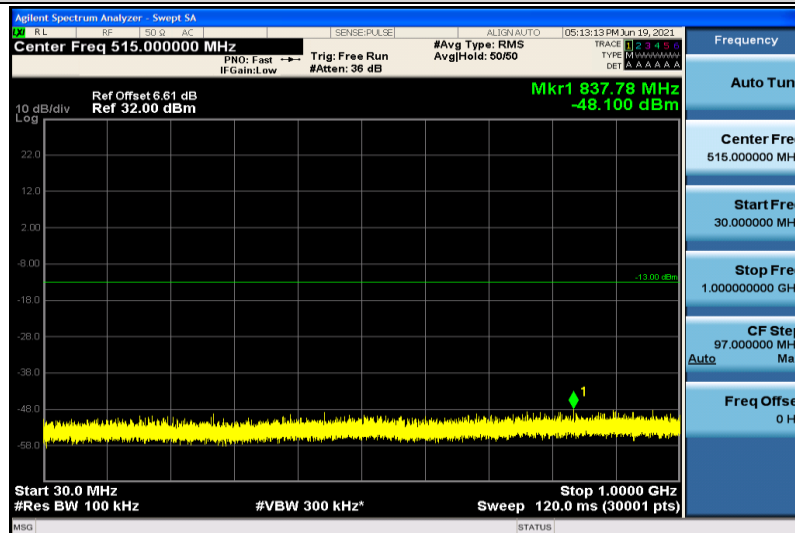
Band25-20MHz-QPSK-26590-1RB#0-30~1000MHz
