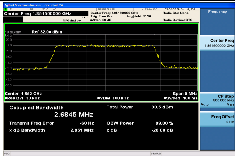
Band2-3MHz-16QAM-18615-15RB#0-2.6845
