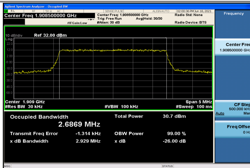
Band2-3MHz-QPSK-19185-15RB#0-2.6869
