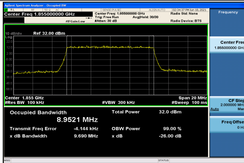
Band2-10MHz-QPSK-18650-50RB#0-8.9521
