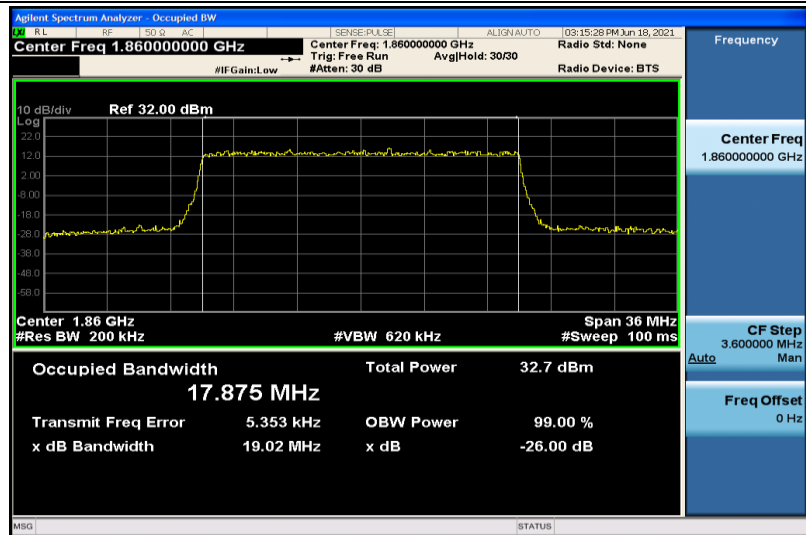
Band2-20MHz-QPSK-18700-100RB#0-17.875
