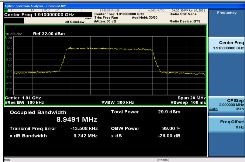
Band25-10MHz-QPSK-26640-50RB#0-8.9491
