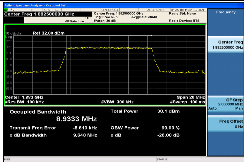
Band25-10MHz-QPSK-26365-50RB#0-8.9333
