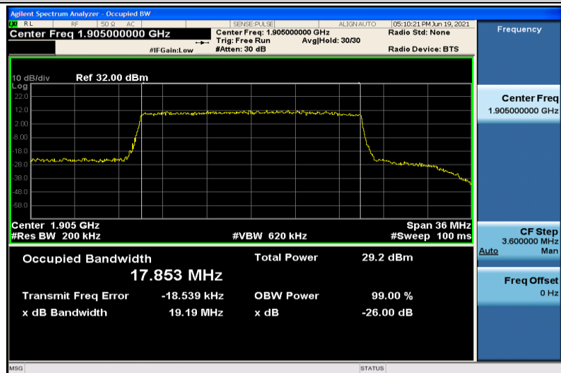
Band25-20MHz-QPSK-26590-100RB#0-17.853
