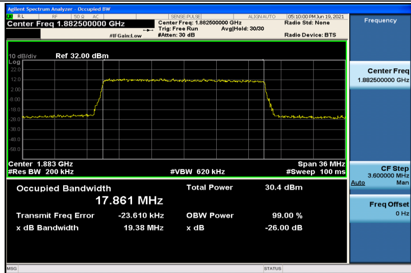
Band25-20MHz-QPSK-26365-100RB#0-17.861
