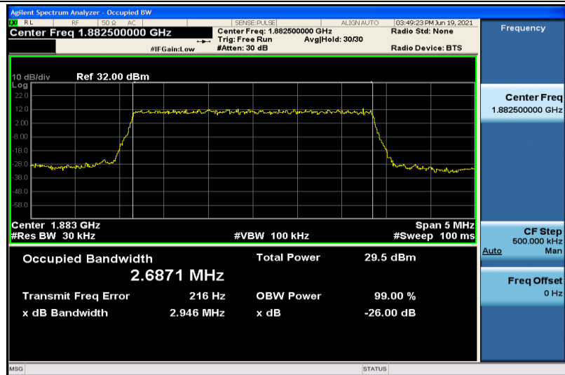
Band25-3MHz-QPSK-26365-15RB#0-2.6871
