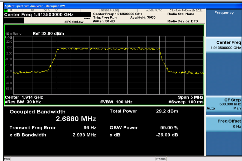
Band25-3MHz-QPSK-26675-15RB#0-2.6880
