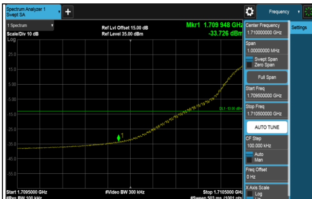
1RB (1715MHz)
