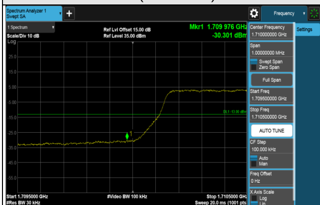
1RB (1711.5MHz)
