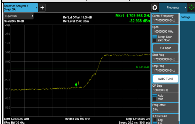
1RB (1711.5MHz)
