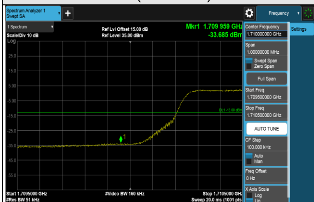
1RB (1712.5MHz)
