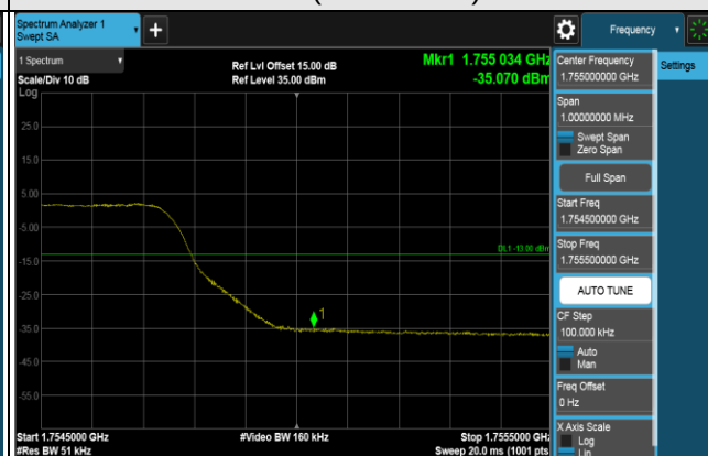
1RB (1752.5MHz)
