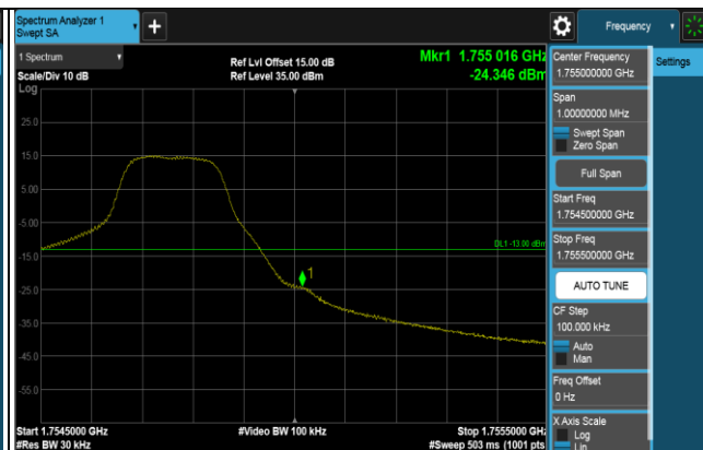
1RB (1753.5MHz)
