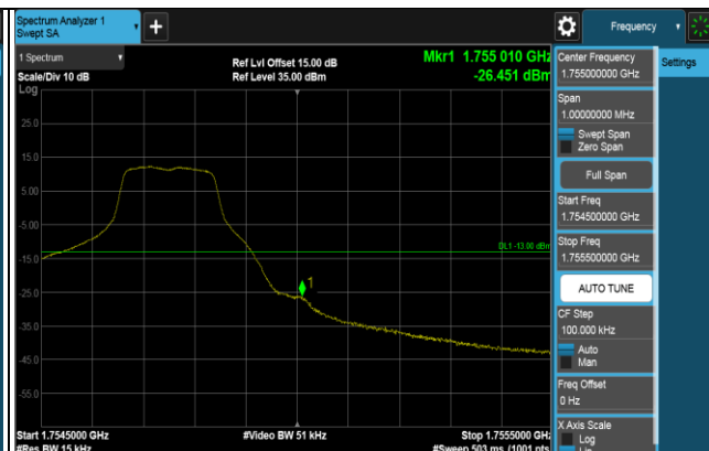
1RB (1754.3MHz)
