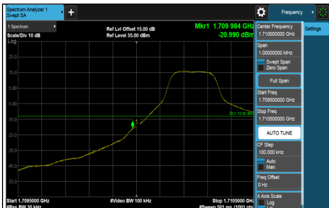
1RB (1711.5MHz)
