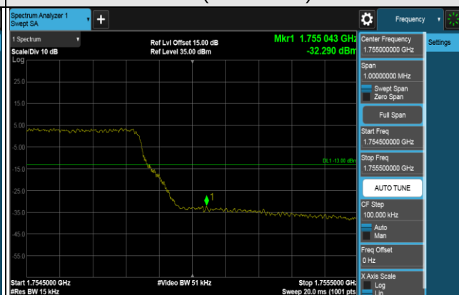
1RB (1754.3MHz)
