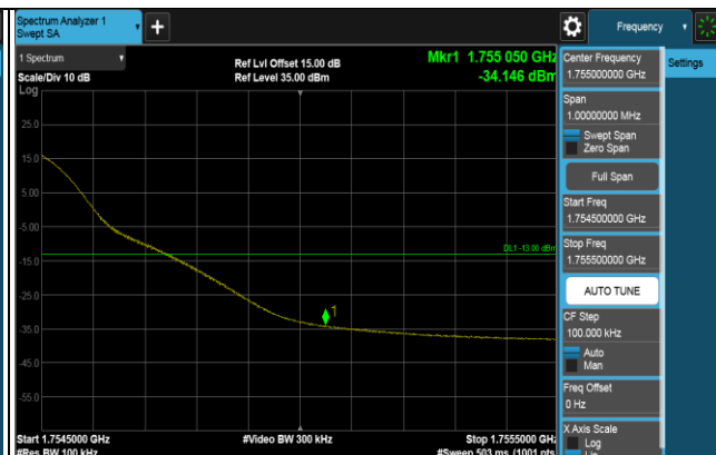
1RB (1750MHz)
