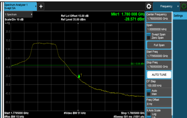
1RB (1779.3MHz)
