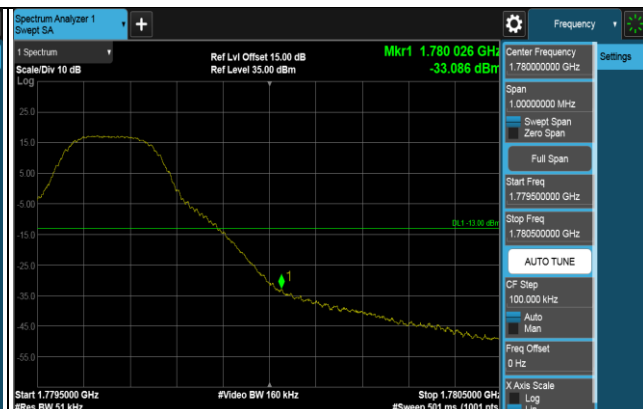
1RB (1777.5MHz)
