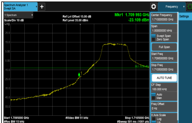
1RB (1710.7MHz)
