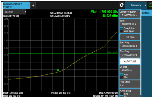
1RB (1715MHz)
