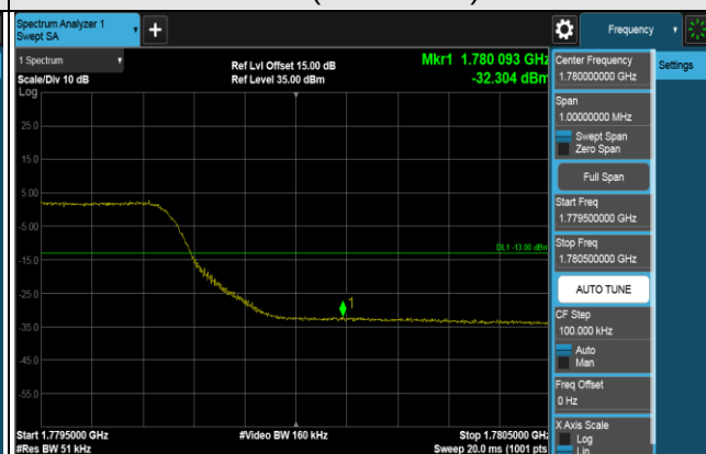
1RB (1777.5MHz)
