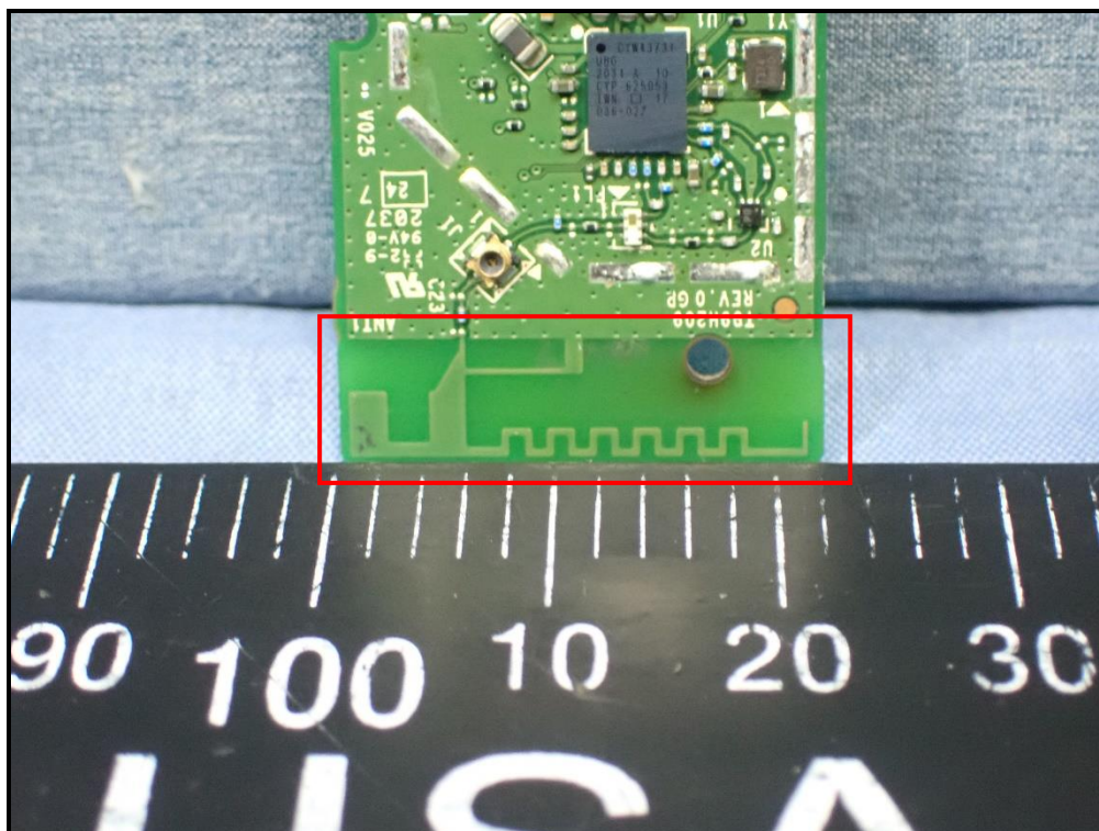
Antenna
