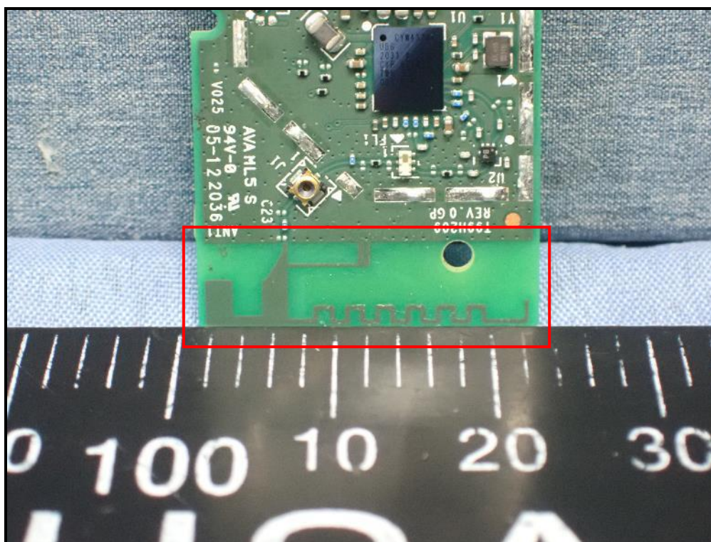
Antenna
