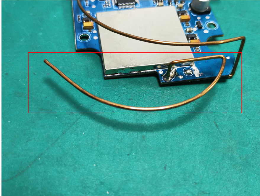
2.4GHz Antenna
