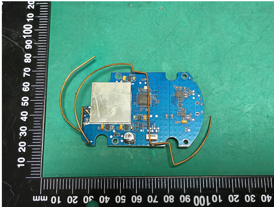
900MHz Antenna
