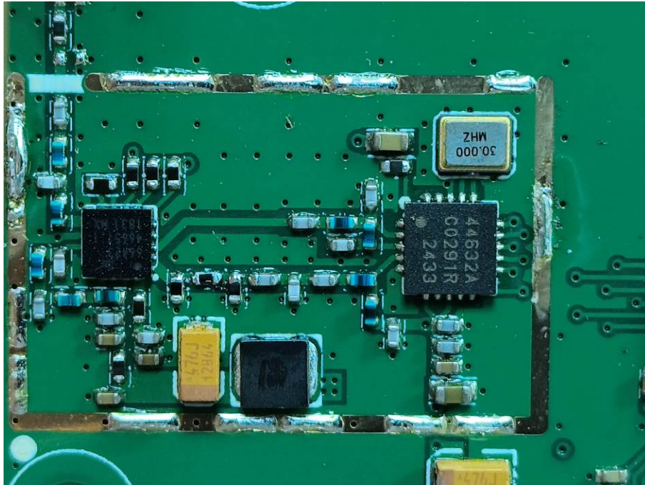
900M ANT
