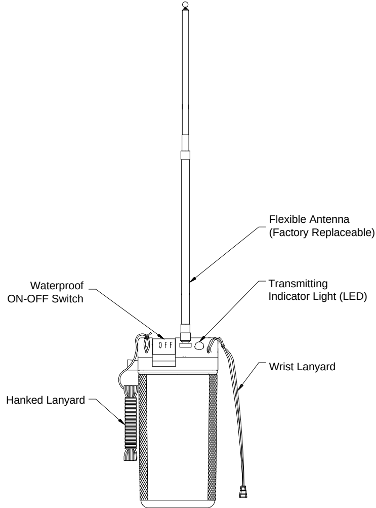
Figure 1: ACR Mini B300™ EPIRB
