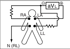
aV L lead
