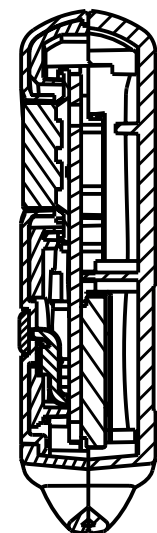
SECTION A-A
